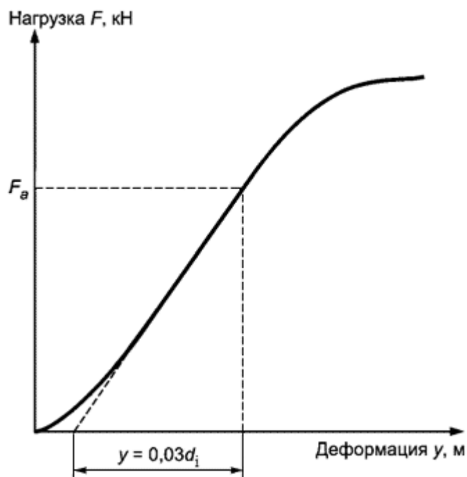
Рисунок В.1 - Кривая "нагрузка-деформация"
